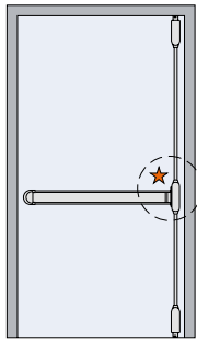
2-punts- vergrendeling
