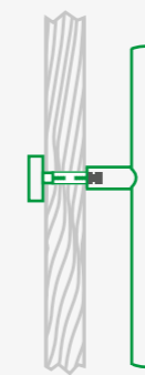
D) Enkelzijdige montage door en door met Thermoshield (type 6011-93)
